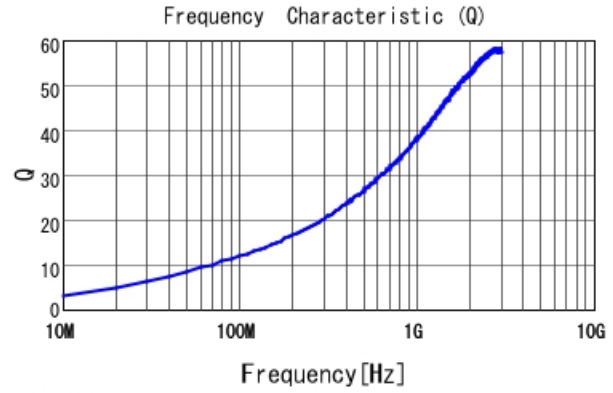
■ LQG15HN3N3S02 Q
