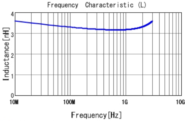
■ LQG15HN3N3S02 L
