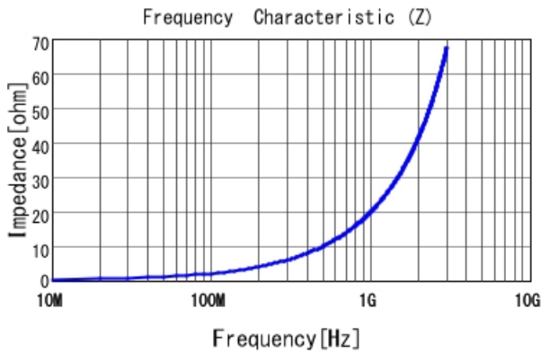
■ LQG15HN3N3S02 |Z|
