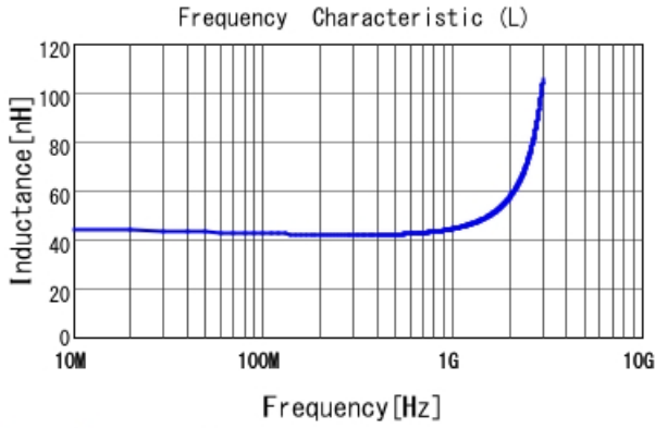
LQW15AN43NJ00 L
