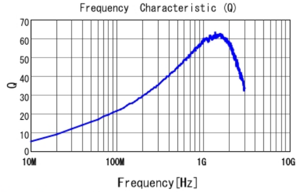
LQW15AN43NJ00 Q
