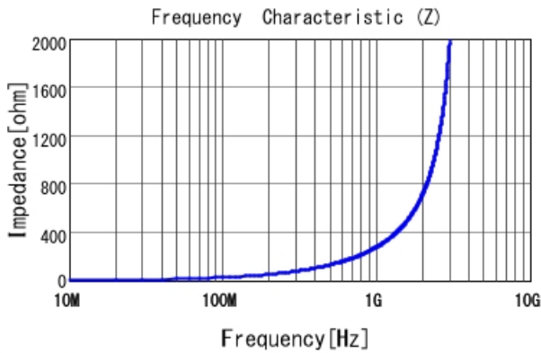
LQW15AN43NJ00 |Z|
